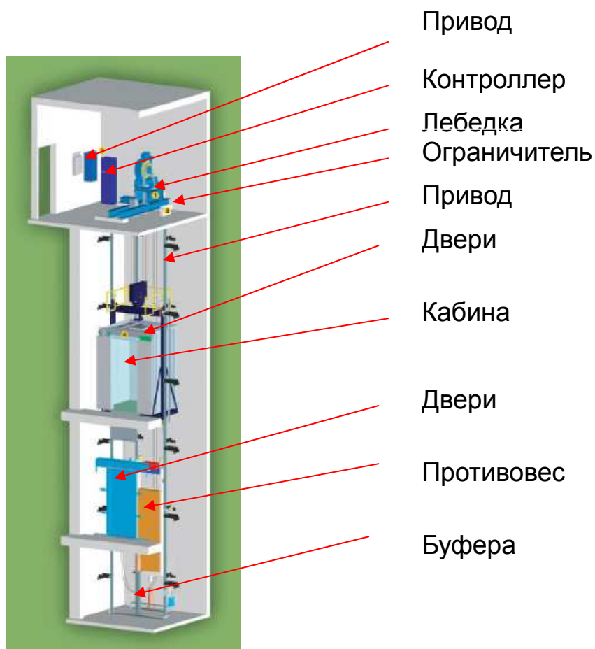
Рис.1 Общий вид лифта
