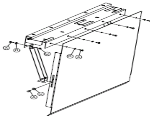
Рис.15. Фартук.
