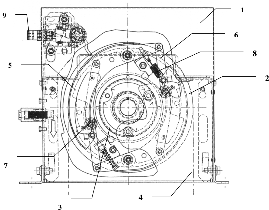
Рис. 18. Ограничитель скорости.
