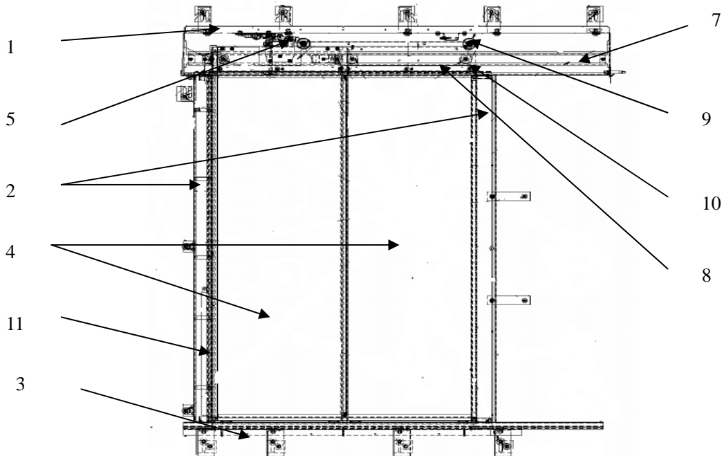
Рис.21. Дверь шахты.
