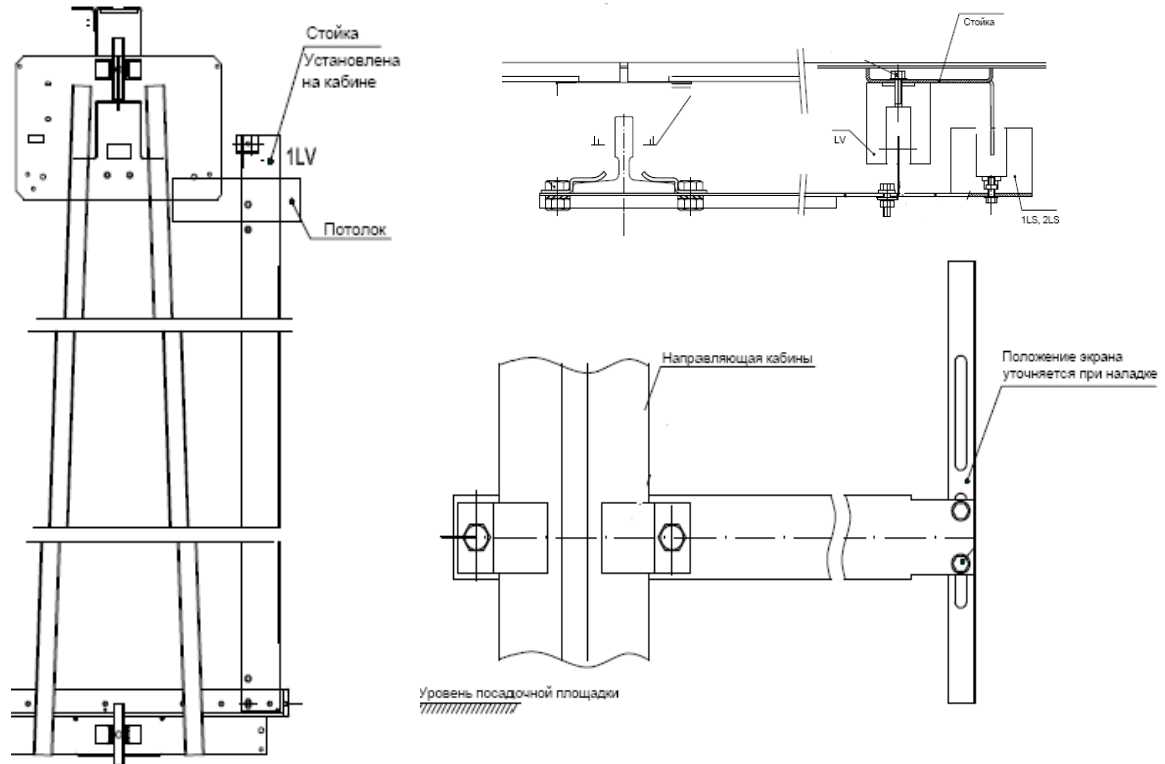
Рис. 24. Система позиционирования с оптическими датчиками LV.
