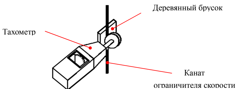
Рис.28. Измерение скорости срабатывания ограничителя скорости при помощи тахометра.
