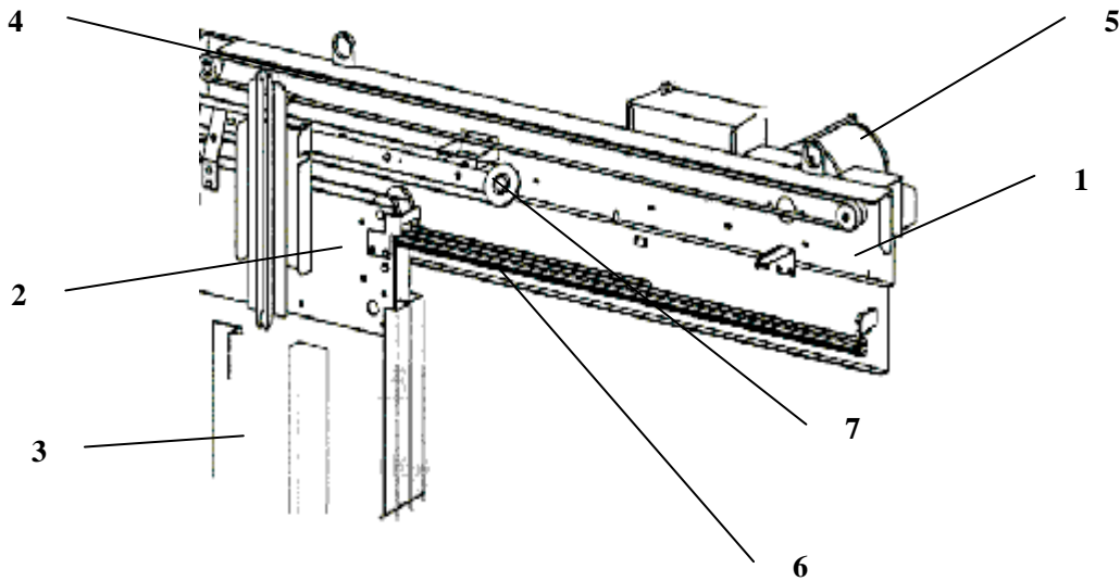
Рис.14. Двери кабины.
