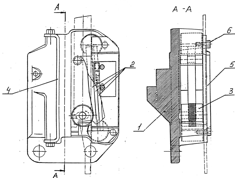
Рис. 16. Ловители.
