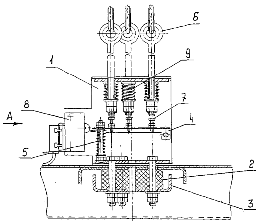
Рис. 9. Устройство контроля слабины и подтягивания канатов (СПК) для подвески 1:1.
